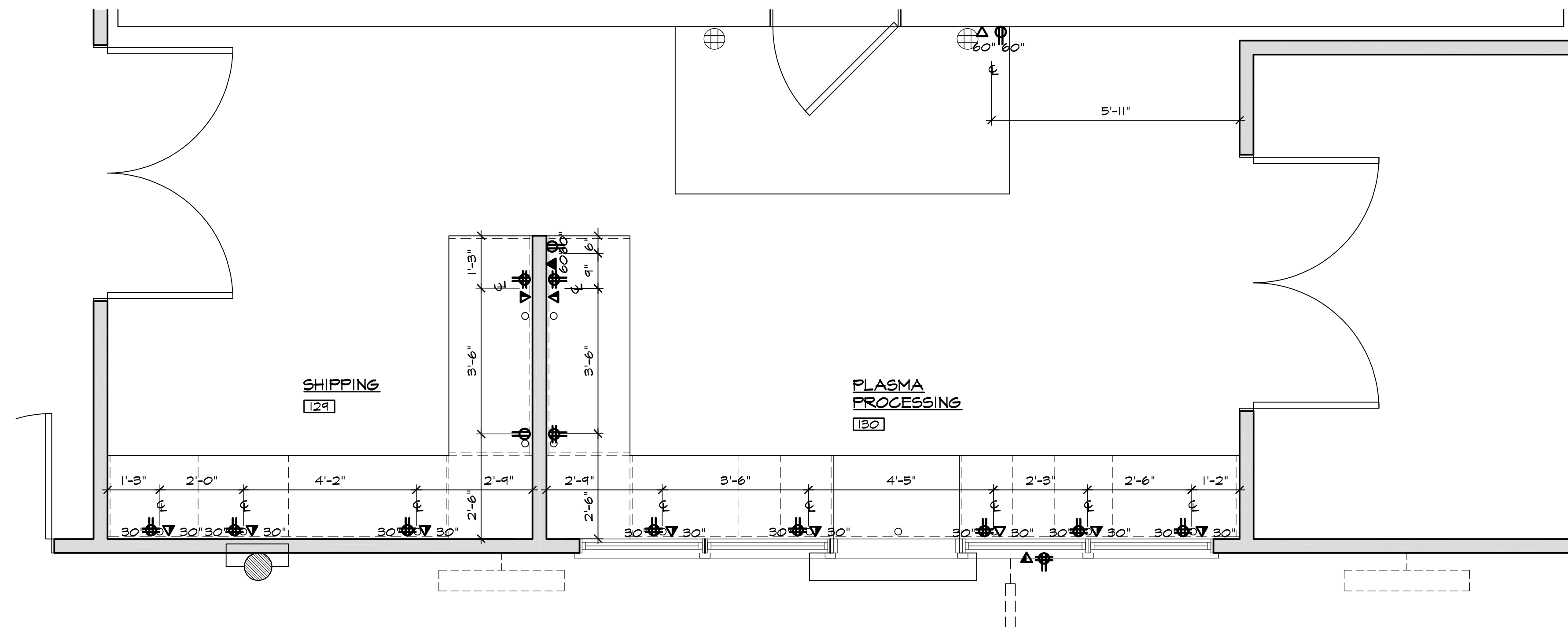
ELECTRICAL OUTLET MOUNTING DIAGRAM, TYP SCALE: N.T.S.
