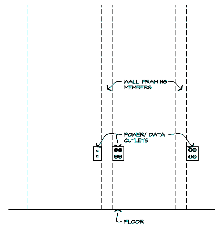
ELECTRICAL OUTLET MOUNTING DIAGRAM, TYP SCALE: N.T.S.
