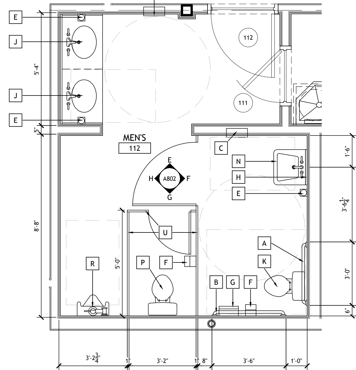
2 MEN'S - 112 A802 SCALE: 3/8" = 1'-0"
