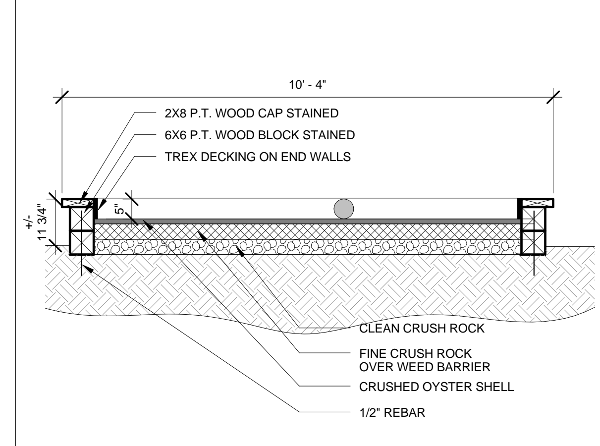
1 BOCCO COURT SECTION SCALE: 1/2" = 1'-0"
