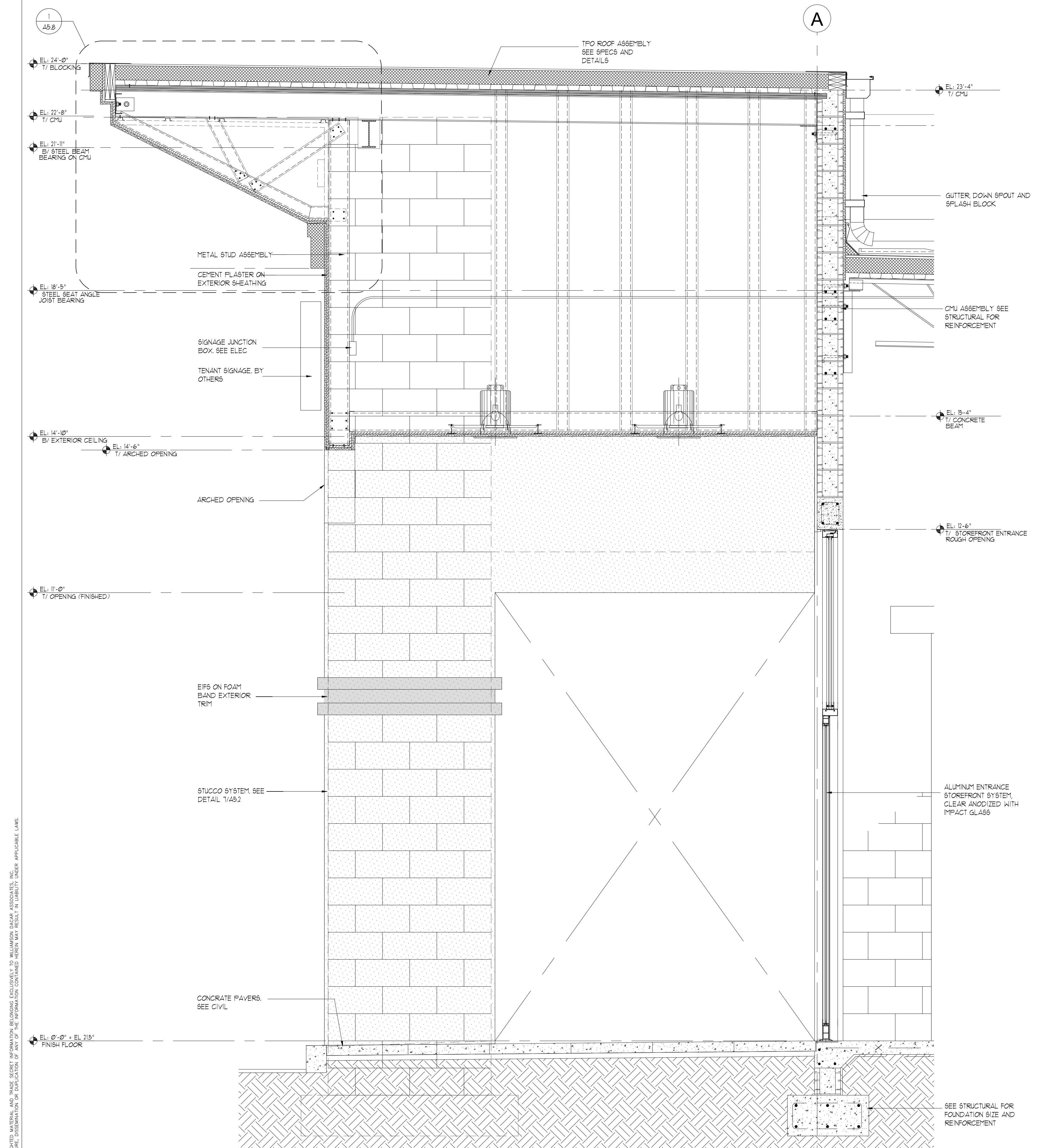
1 A5.4 WALL SECTION SCALE: 3/4" = 1'-0"
